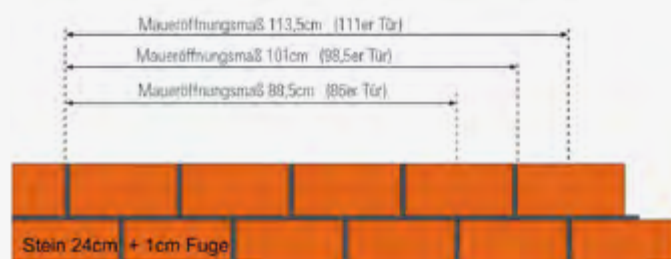
Baurichtmaße als Maßketten in der Breite
